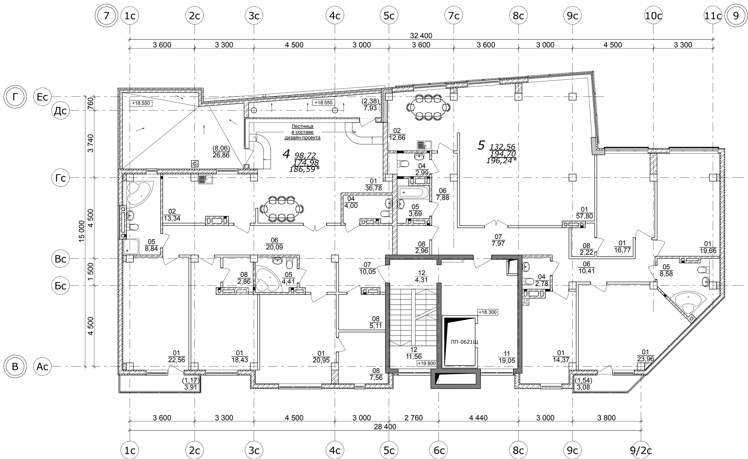
Экспликация помещений
