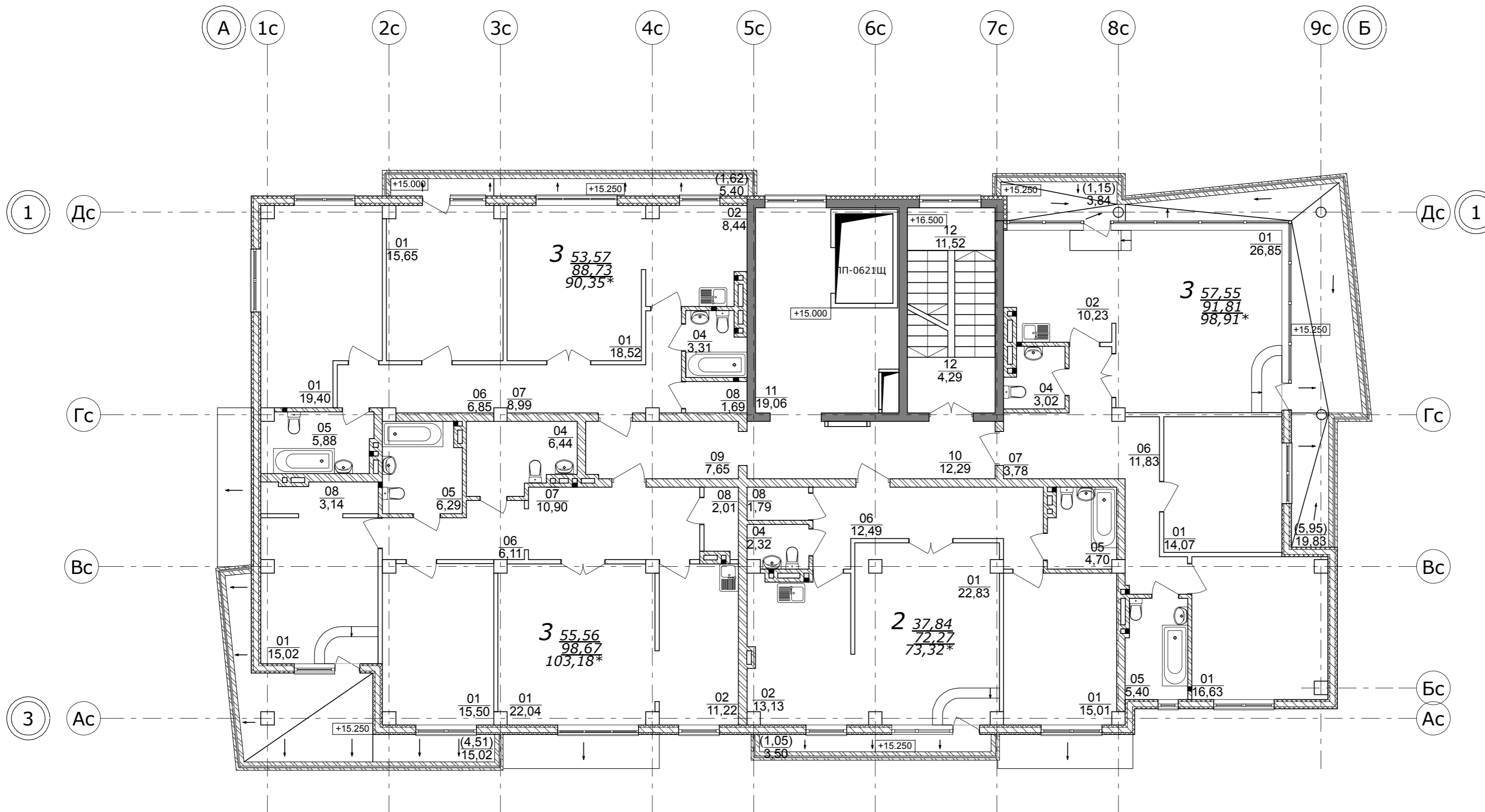
Экспликация помещений
